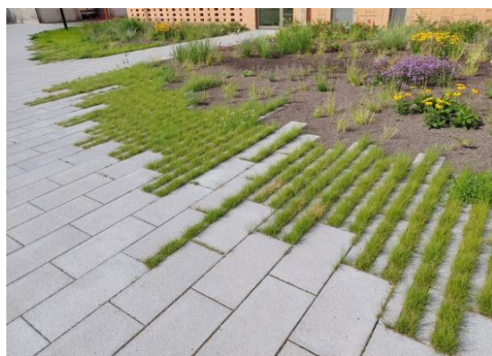
Princip dlažby proluté se záhony
