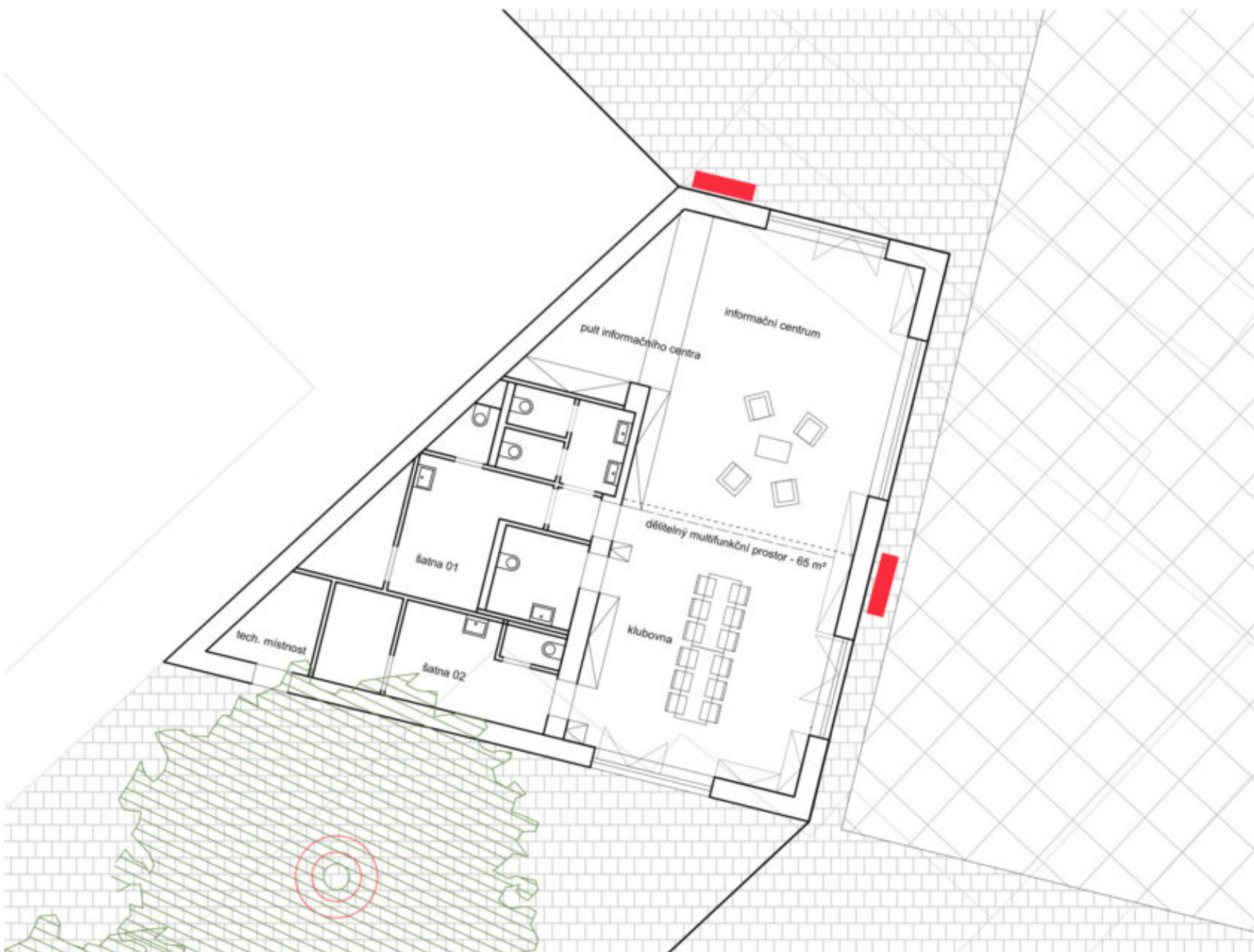
schématický půdorys varianty
